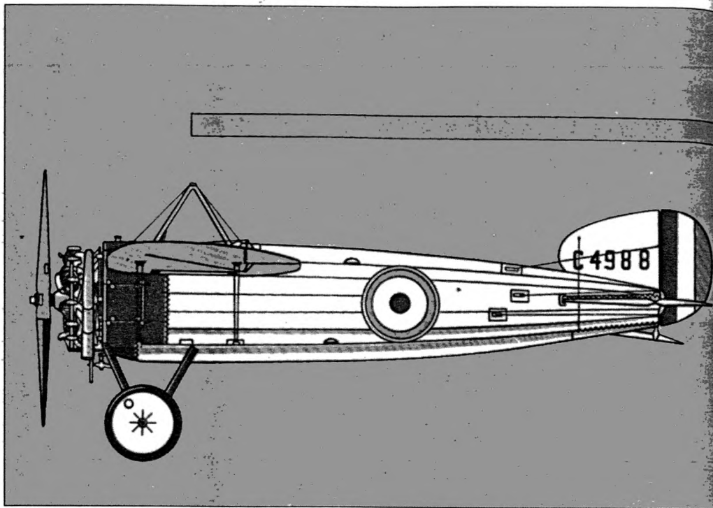
Avión Bristol M1C. El ejemplar de la ilustración es una réplica de escala 1:1 en estado de vuelo y pertenece a la colección de aeronaves del Museo Nacional Aeronáutico de Chile.
