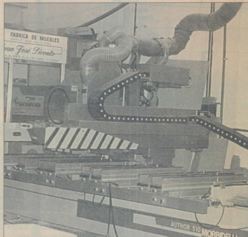
Máquina punto a punto con control numérico. Este es uno de los elementos de los equipos de avanzada con los que cuenta la empresa.
