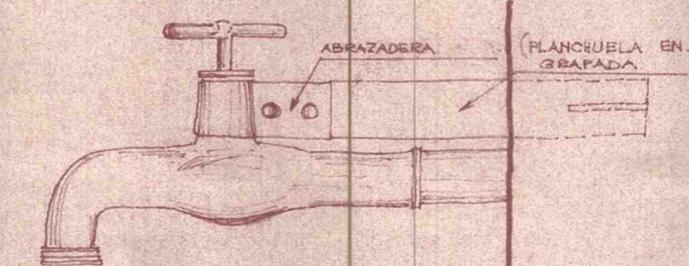
CANILLA SURTIDORA
