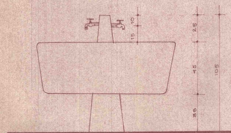
VISTA
