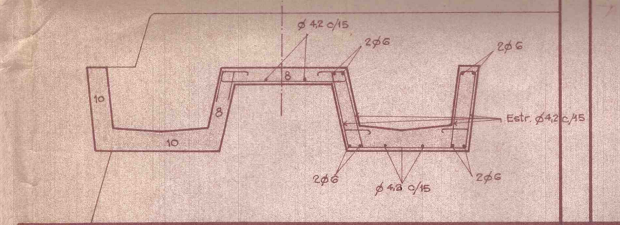
CORTE BB
