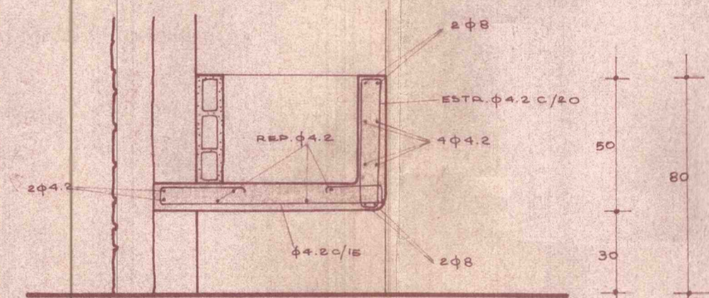
CORTE BB
