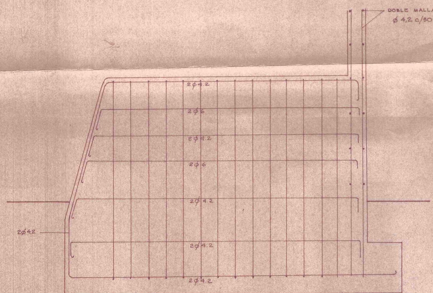
CORTE CC
