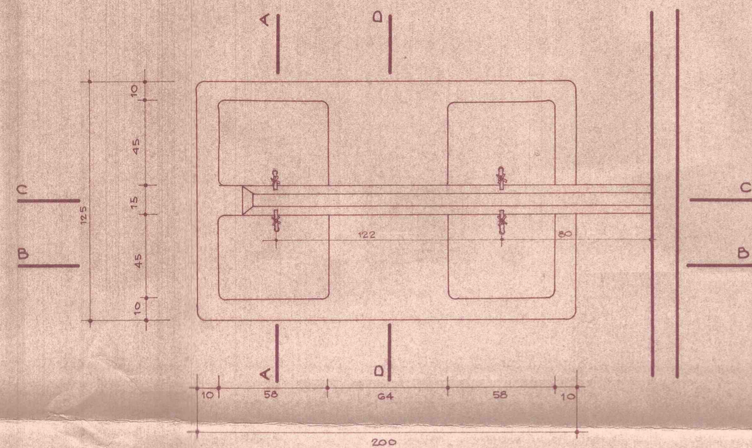
PLANTA
